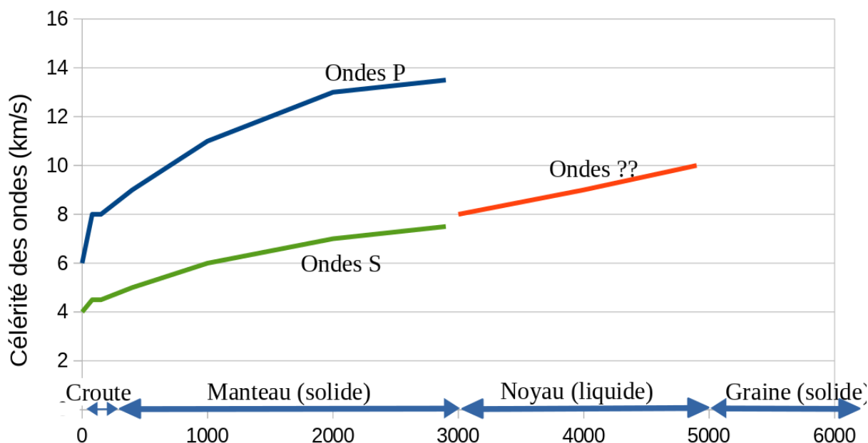
Profondeur de la Terre mesurée à partir du sol (km) Graphe : célérité des différents types d'onde dans la structure terrestre (d'après données planet-terre.ens-lyon.fr)
