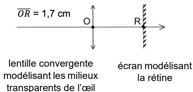
Figure 2 : Montage optique modélisant l'œil
