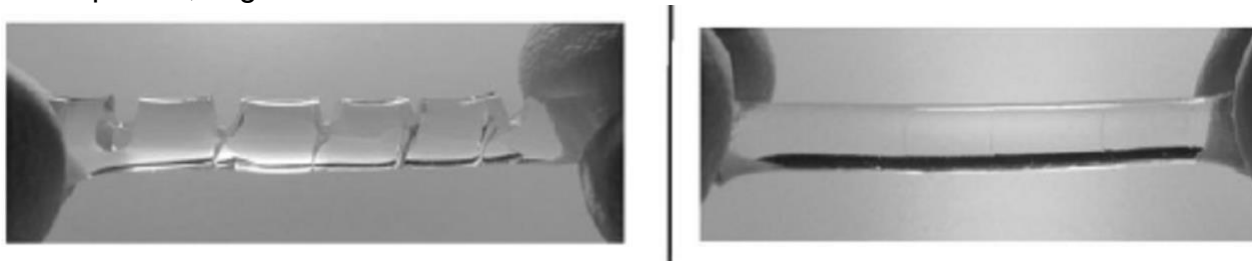
Figure 1: à gauche, un hydrogel coupé et à droite ce même hydrogel autocicatrisé D'après publication de K.Haraguchi https://onlinelibrary.wiley.com/doi/abs/10.1002/marc.201100248
