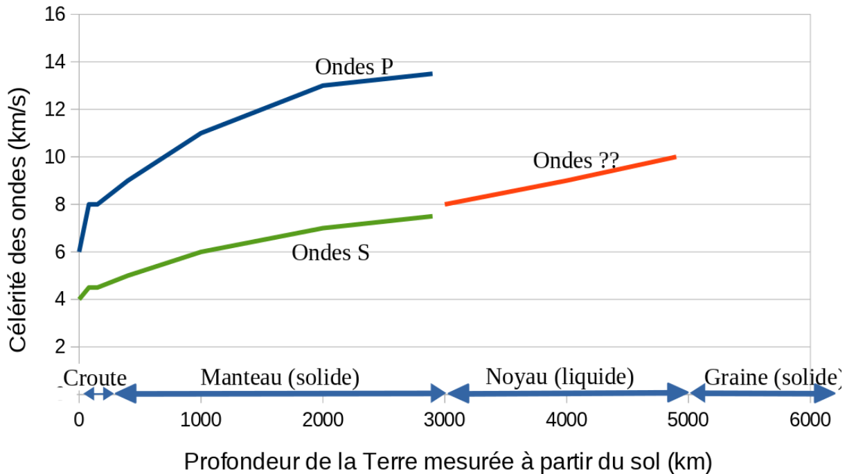
Profondéur de la Terre mesurée à partir du sol (km) Graphé : célérité des différents types d'onde dans la structure terrestre (d'après données planet-terre.ens-lyon.fr)
