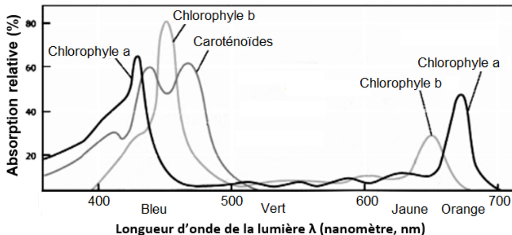
Spectres d'absorption des chlorophylles a et b ainsi que des caroténoïdes (d'après http://www.cima.ualg.pt/l )
