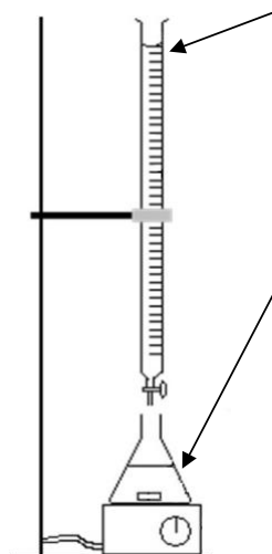
Schéma du montage du titrage
