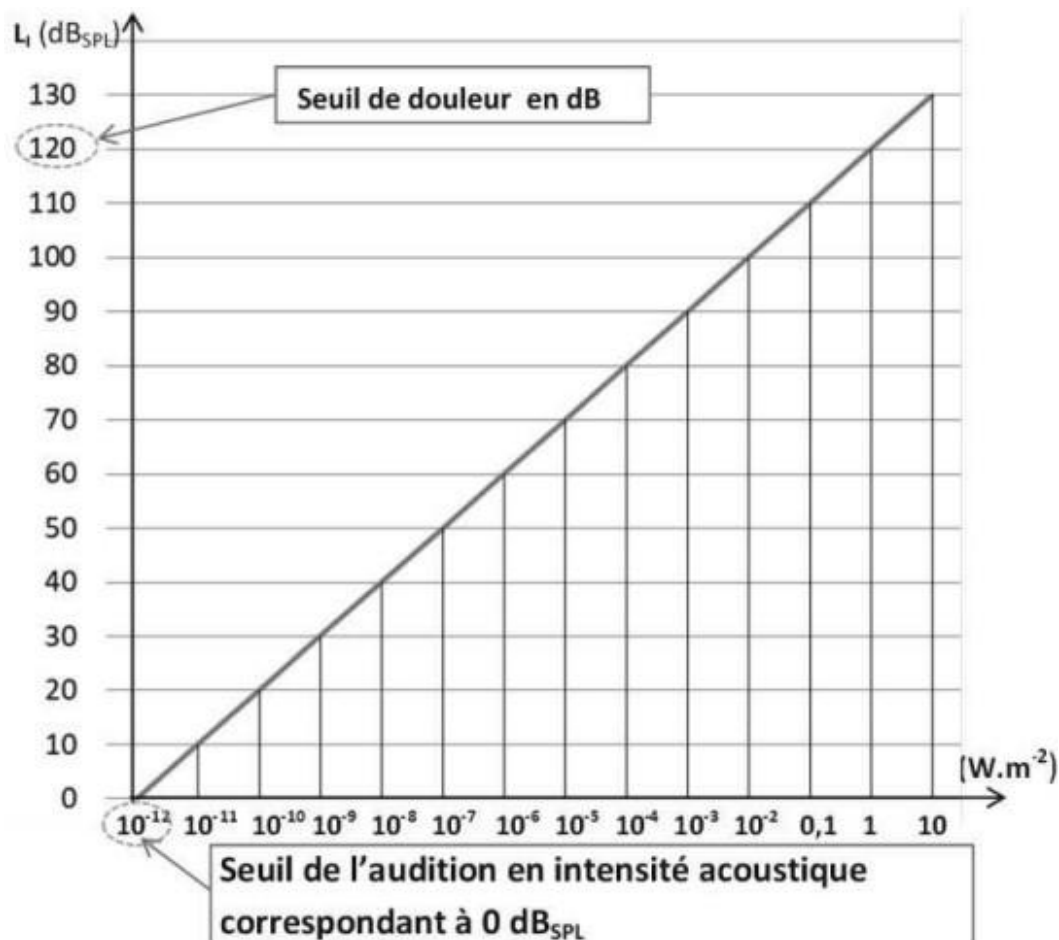
Document 3 – Évolution du niveau d'intensité sonore (en dB) en fonction de l'intensité sonore (en \text{W.m}^{-2} )
