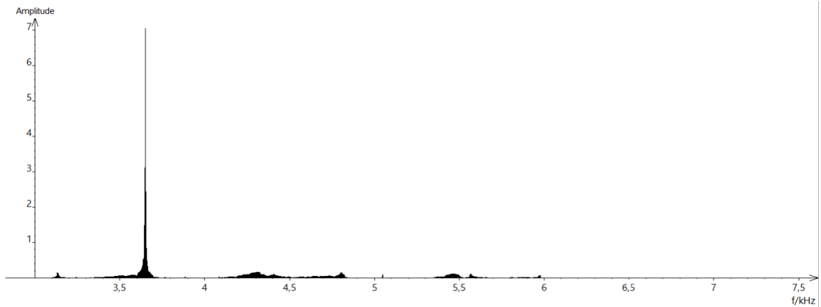
Spectre du son obtenu avec le marteau 2
